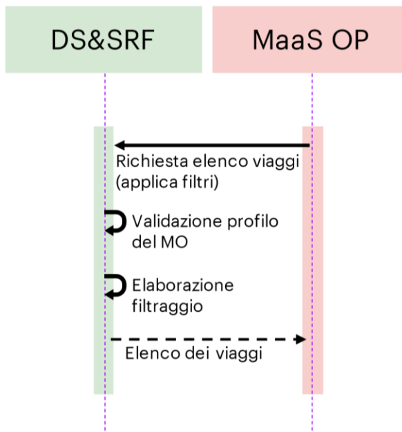
Figura 1 - Recupero elenco dei viaggi per i Maas Operator
