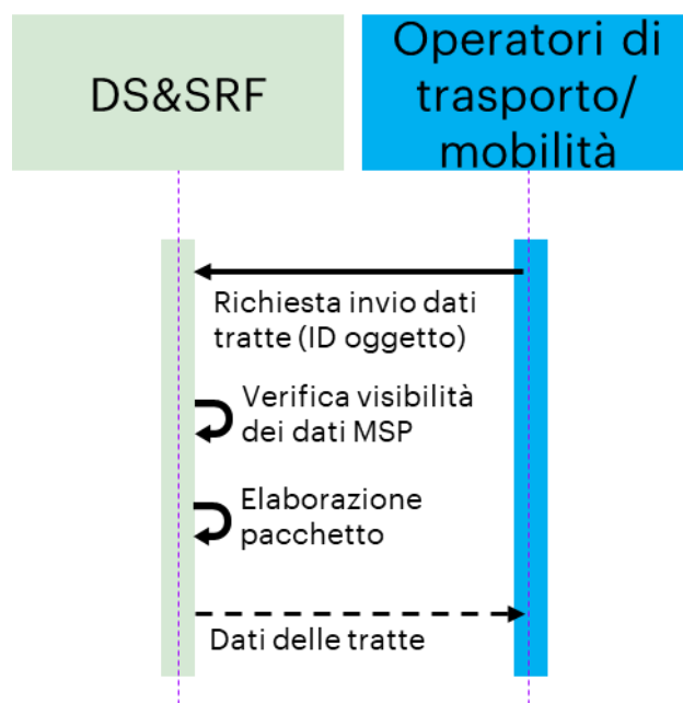
Figura 4 - Recupero informazioni sulle tratte di competenza degli operatori di trasporto/mobilità
